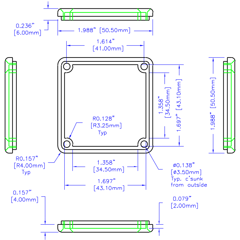
LID
