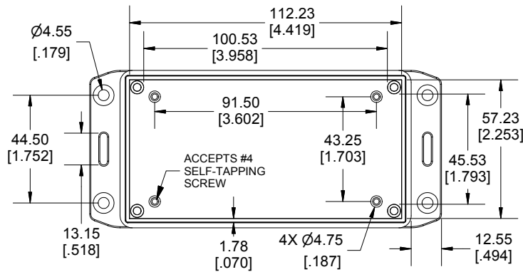
INSIDE LID
