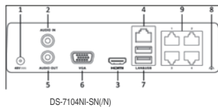
DS-7104NI-SN(/N)
