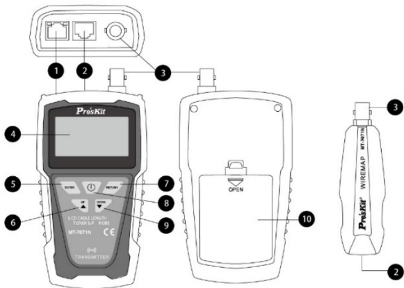
發射器及測試遠端產品示意圖
