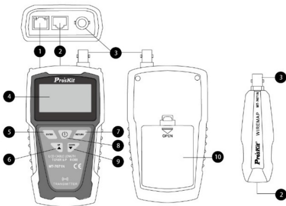
发射器及测试远程产品示意图
