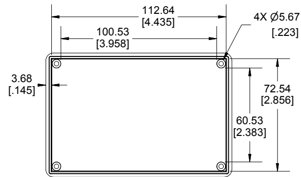
INSIDE LID
