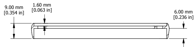
OPEN BEZEL
