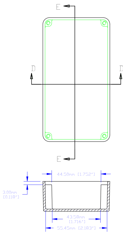
D-D (1:1)
