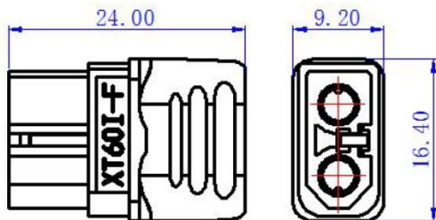
XT60I-F
